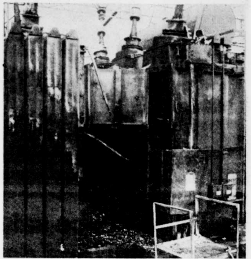
Le transformateur incendié d'Hydro-Québec d'où s'est échappée l'huile contenant des BPC.
