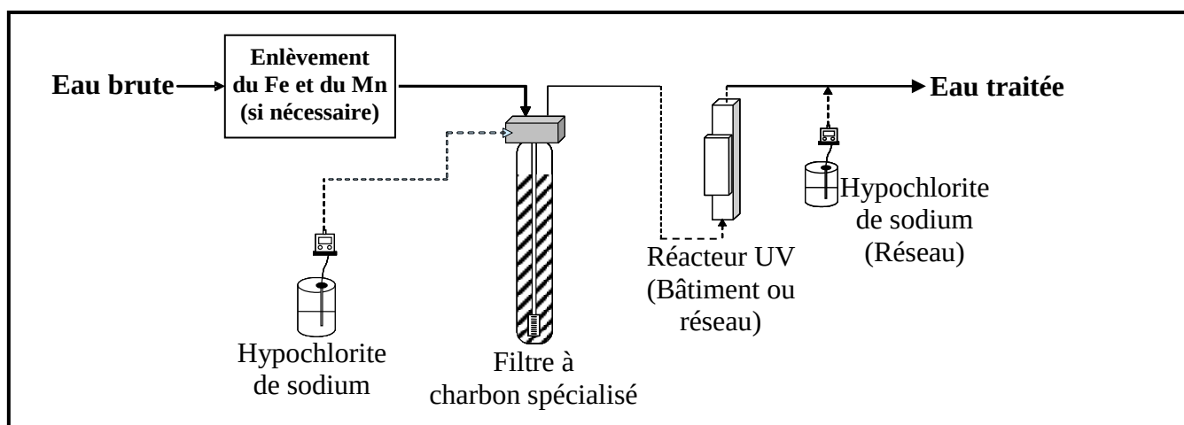
Figure 8 Schéma d'écoulement basé sur une filtration sur charbon spécialisé pour l'élimination des sulfures (le chlore avant le filtre ne sert qu'à la régénération du charbon spécialisé)
