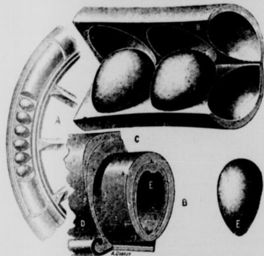
Détails du pneumatique "Invictus" A, pneu monté; B, section de chambre ouverte; C, coupe transversale de la chambre; D, enveloppe; E, oeuf.
