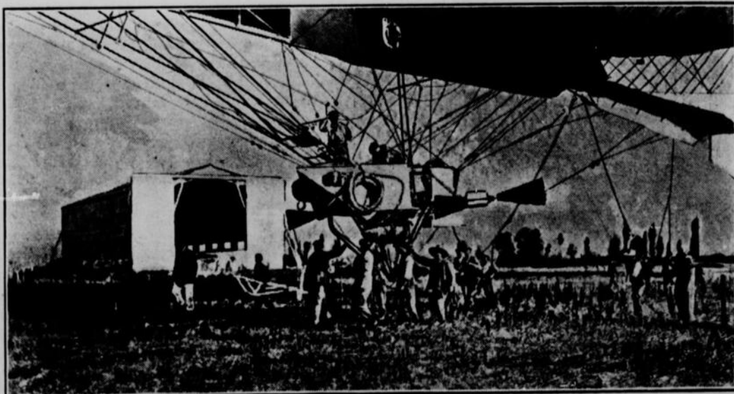
Détails de la nacelle et de la machinerie du "Lebaudy No 2"
