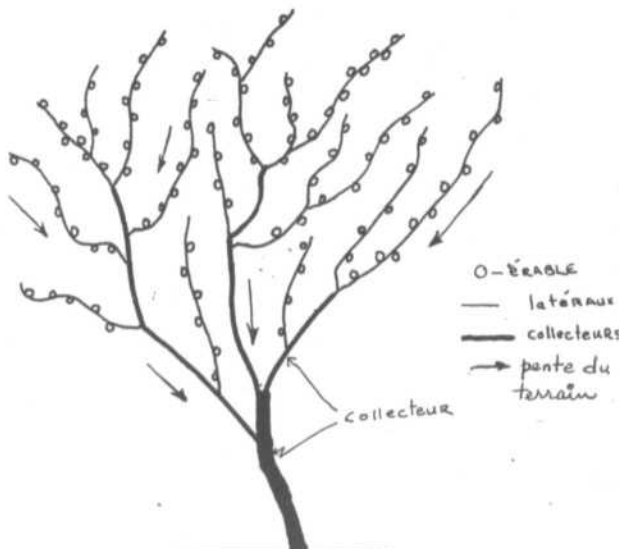
Représentation schématique d'une installation de collecte de sève avec tubulure et pompe à vide.
