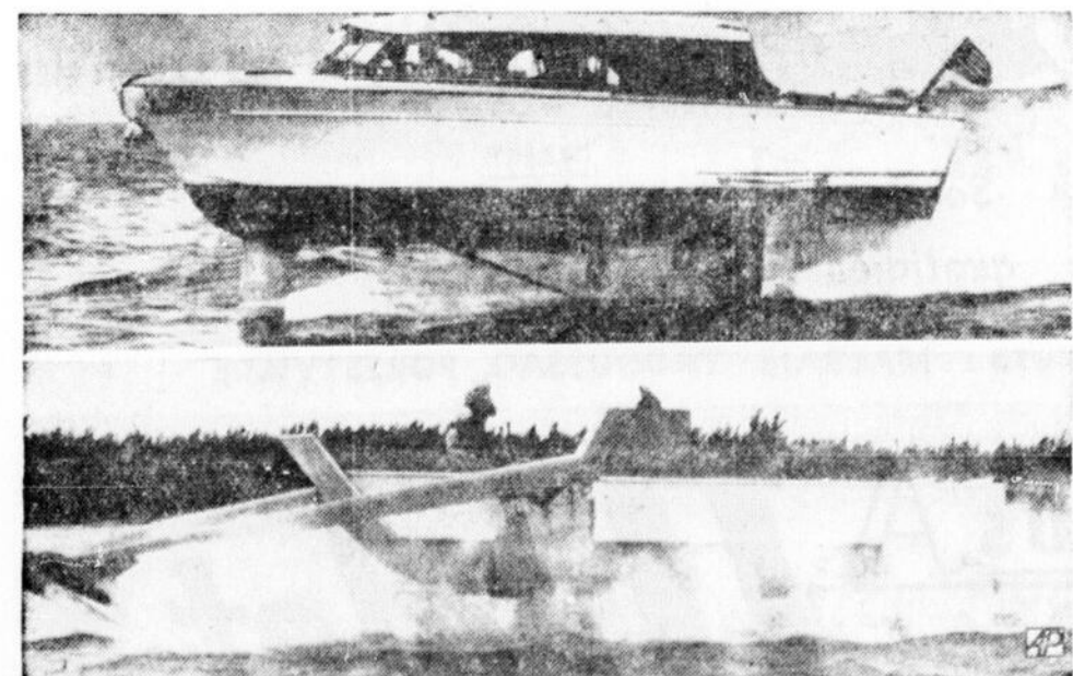
ESSAI DE NAVIRES SUR PATTES : Deux navires "volants", le "Sea Legs" (en haut) et le "Halobates", sont mis à l'essai par la marine américaine. Ils peuvent aller à une vitesse de plus de 25 milles à l'heure. Le "Sea
