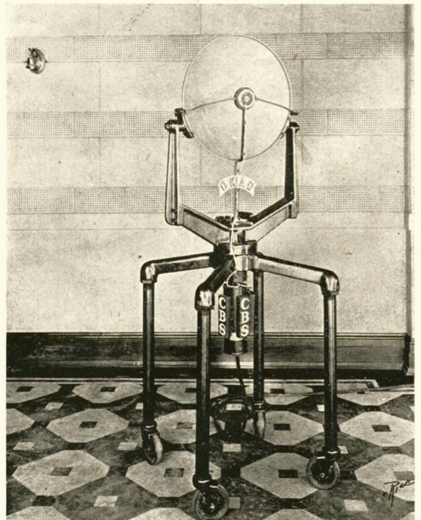
Le microphone parabolique du poste CKAC
