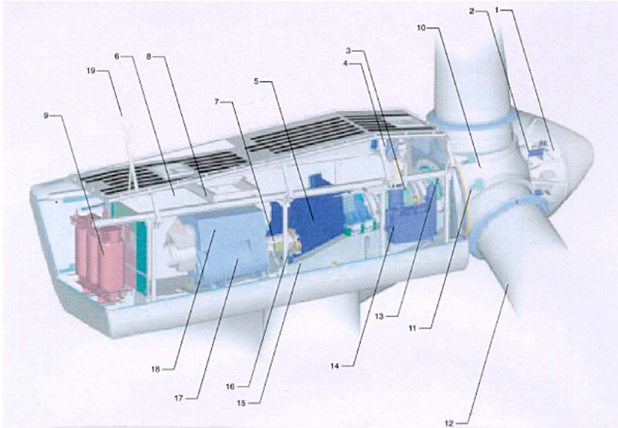
FIGURE 2 : DÉTAILS DES ÉQUIPEMENTS CONTENUS DANS LA NACELLE
