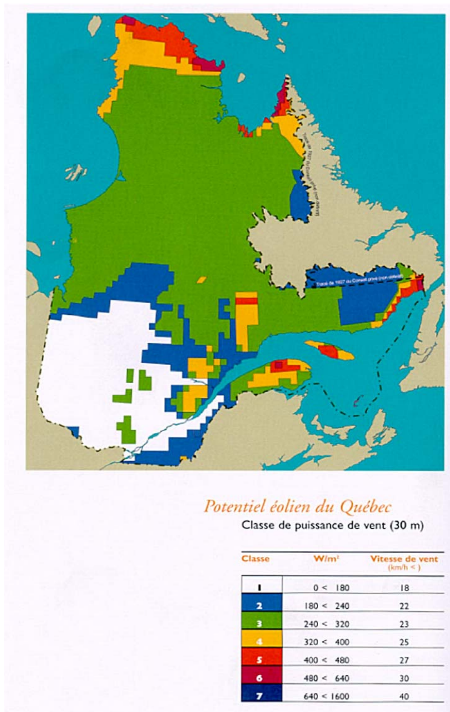
FIGURE 3 : RÉGIONS OFFRANT UN POTENTIEL ÉOLIEN
