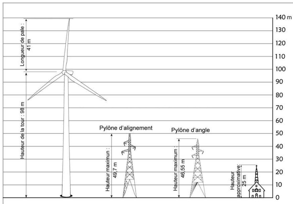
Figure 4 La hauteur des éoliennes et des pylônes de la ligne de raccordement
