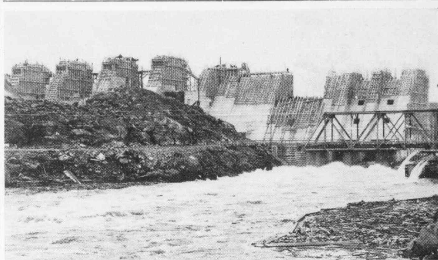
L'AMENAGEMENT DE LA CENTRALE DE CHUTE-A-LA-SAVANNE VA BON TRAIN. — Cette photographie prise vendredi dernier nous donne une excellente idée où en sont rendus les travaux d'aménagement de la centrale hydro-électrique d'Alcan à Chute-à-la-Savanne. Comme le fait voir cette photographie, l'on a commencé à enlever les formes
