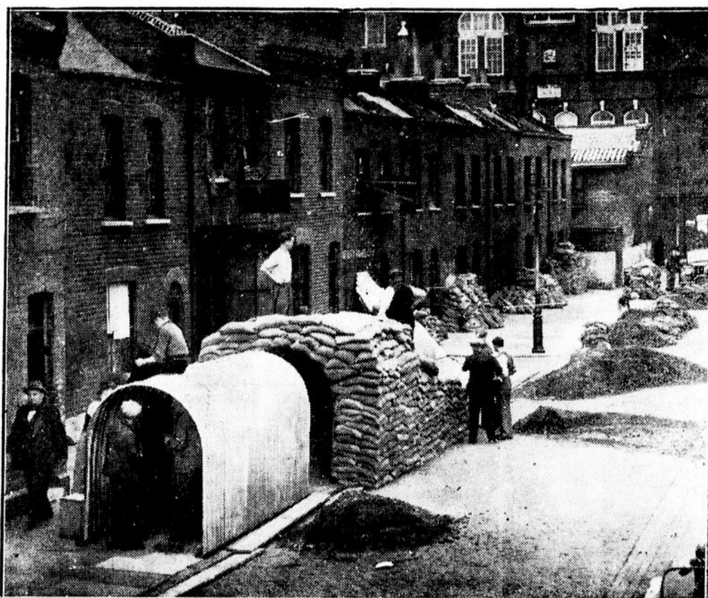
• Dans les quartiers pauvres de Londres, les abris contre les attaques soudaines doivent être construits pour les milliers d'habitants, qui n'ont pas de cours pour construire ces abris. Les "Abris Anderson" en tôle ondulée et avec des sacs de sable sont construits dans les rues.
