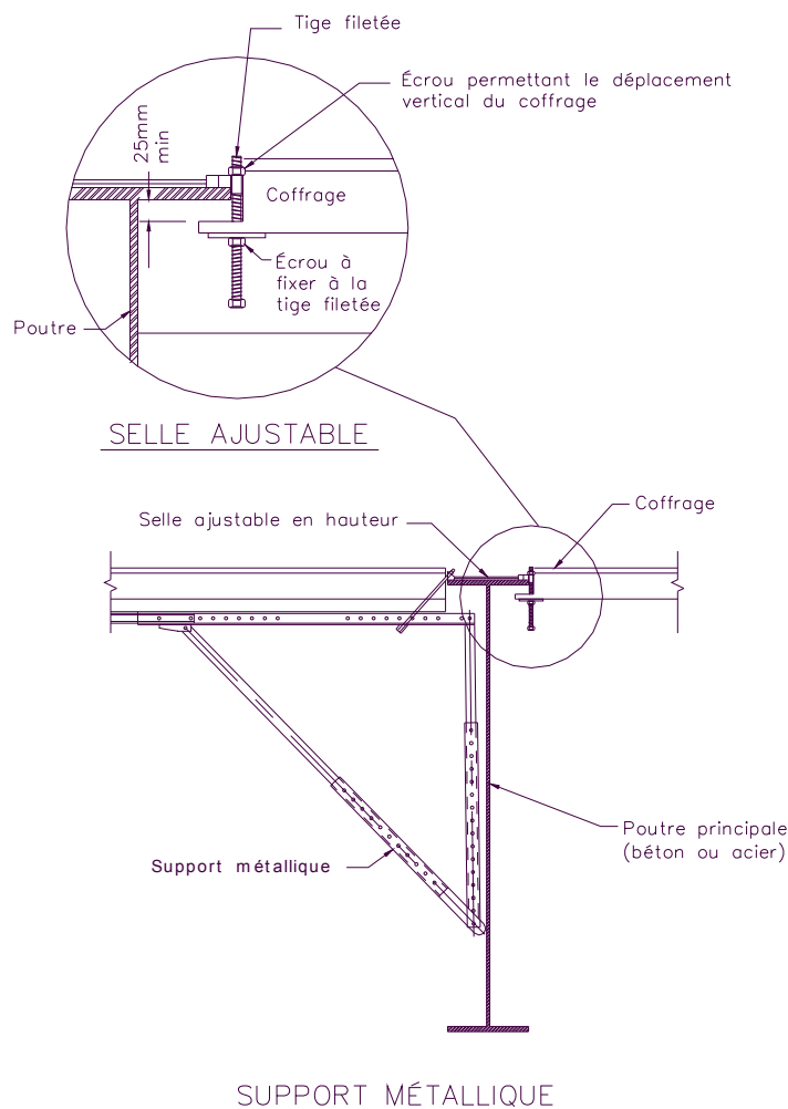
Figure 4.3-4 Support métallique et selle ajustable en hauteur
