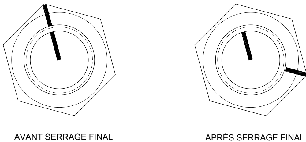
Figure 7.6-1 Exemple de marquage du boulon et de l'écrou pour un serrage final à 1/3 de tour
