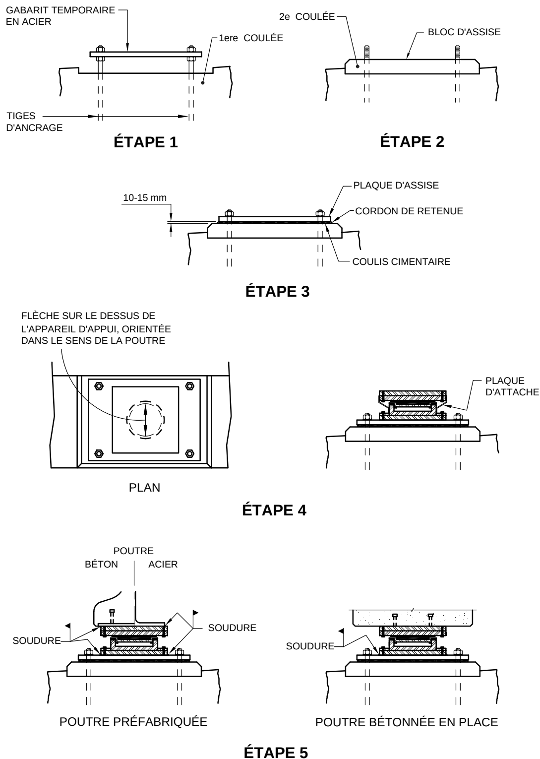
Figure 9.1-2 Étapes de mise en place d'un appareil d'appui à élastomère confiné – exemple
