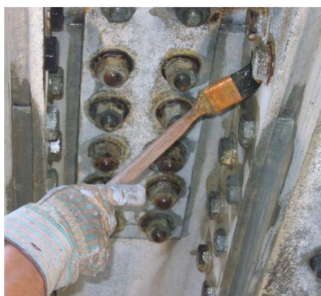
5. Badigeonnage de boulons
