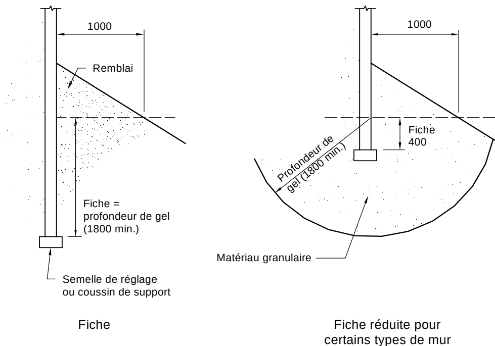
Figure 2.5-3 Profondeur des fondations
