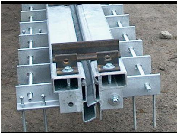
5. Joint de tablier de type HSS
