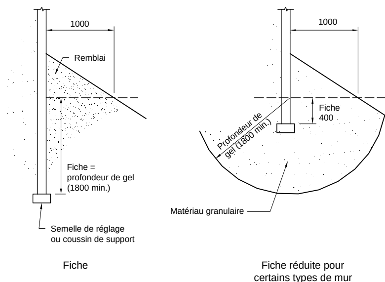
Figure 12.2-1 Profondeur des fondations
