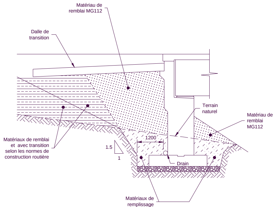
Figure 2.5-4 Remplissage des excavations et mise en place du remblai à proximité d'une culée
