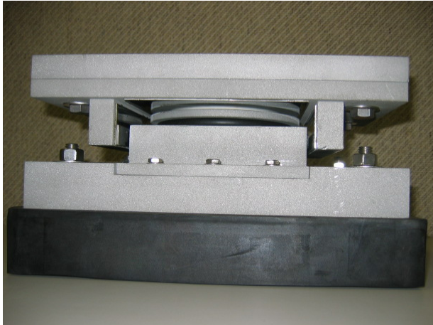
1. Appareil d'appui à élastomère confiné (guidé)
