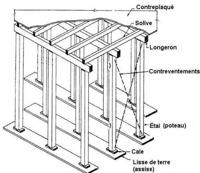
Figure 4.3-7 Terminologie d'un étalement
