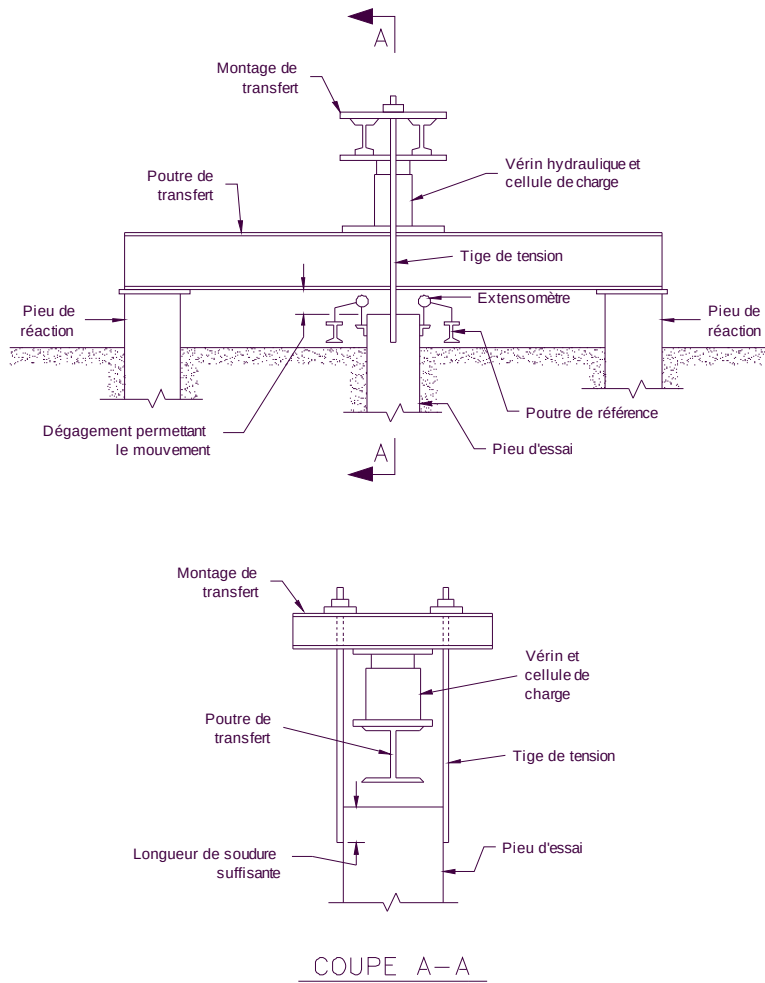
Figure 3.5-4 Montage pour essai en traction – avec un seul vérin
