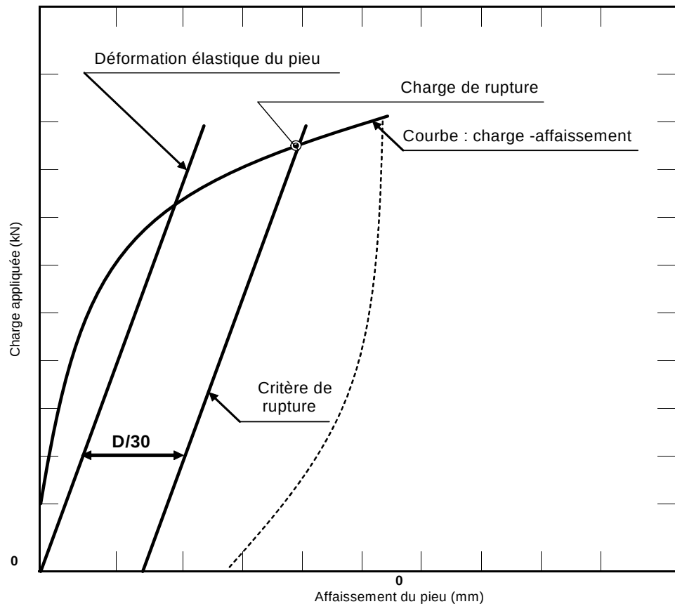
Figure 3.5-8 Représentation d'un graphique « charge – affaissement »
