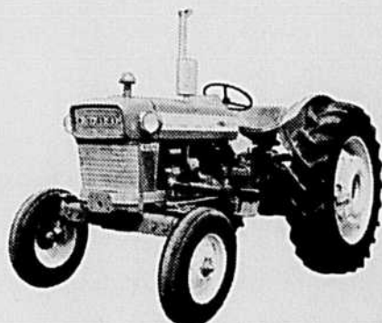
LE NOUVEAU FORD MAJOR 4000. Un tracteur universel de 55 CV* d'une force herculéenne et d'une endurance à toute épreuve, dans une des catégories de puissance les plus demandées. Moteur diesel ou à essence. Démultiplication finale à double réduction. Capacité 3-4 socs.
