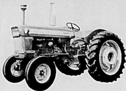
LE NOUVEAU FORD SUPER MAJOR 5000. Un gros tracteur universel à moteur diesel Ford de 65 CV*. Plus de deux tonnes et demi de "muscle" pour effectuer les plus gros travaux sur la plupart des fermes. Confort et manœuvrabilité dans la meilleure tradition Ford. Capacité 4 socs.
