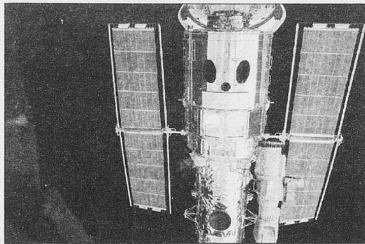
TÉLÉSCOPE — Une superbe vue du télescope Hubble lorsqu'il a été «capturé» par la navette Discovery.
