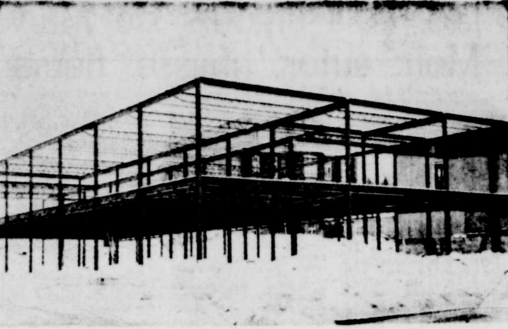
LA STRUCTURE d'acier de l'école des filles de Saint-Thécle a été posée la semaine dernière. Cette photo nous montre une partie de cette construction qui aura plus de deux cents pieds de longueur par une hauteur de deux étages. A l'arrière plan, nous pouvons apercevoir le vieux couvent qui sera démoli. Le droit de l'église paroissiale. Cette structure comprend l'une des plus longues poutres d'acier jamais coulées pour une construction de ce genre.
