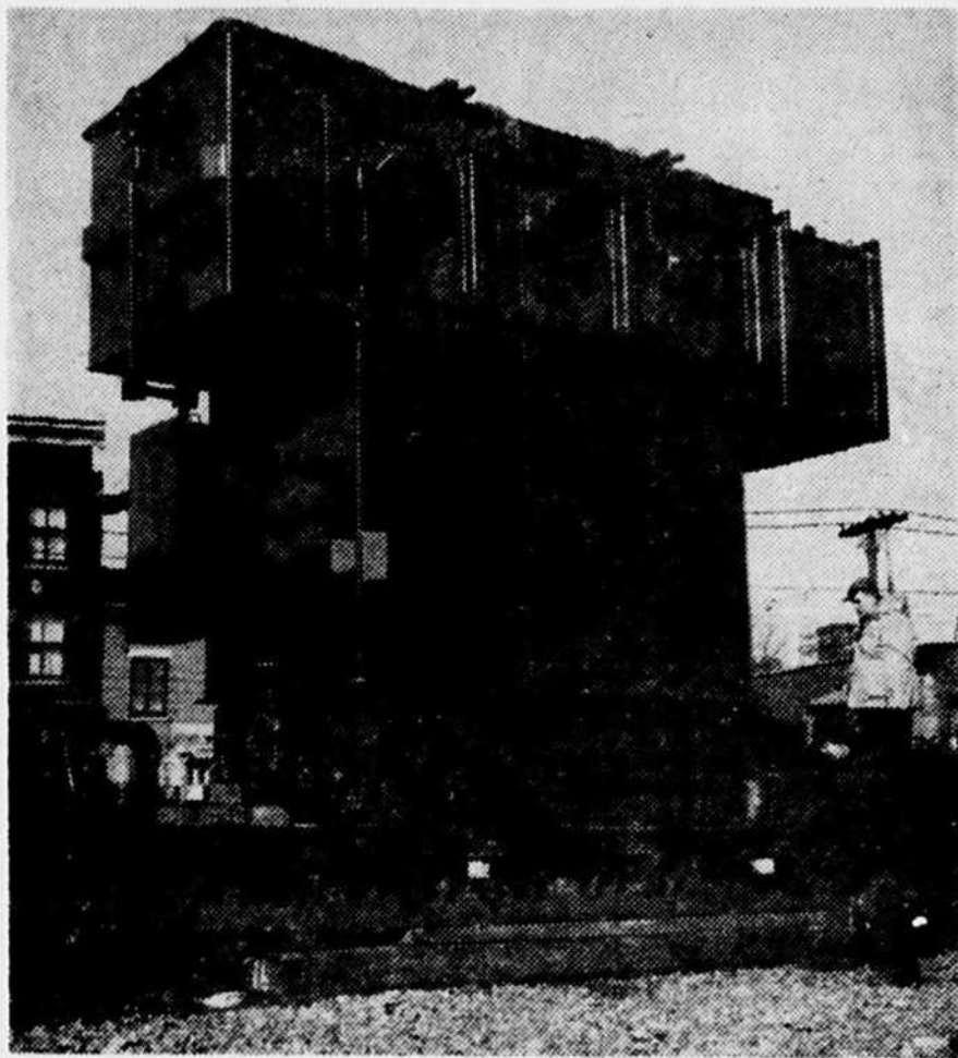
TRANSFORMATEUR GEANT — Ce transformateur géant, destiné à la sous-centrale de l'Hydro-Québec, située sur la rue Guy, vient de Hamilton, Ontario, et a été transporté à Montréal sur un wagon plateforme surbaissé du Canadien National. Ce transformateur pèse 75 tonnes et le train spécial qui l'a conduit à Montréal a circulé à une vitesse de 25 milles à l'heure sur lignes droites et à 10 milles dans les courbes. (Photo Canadien National)
