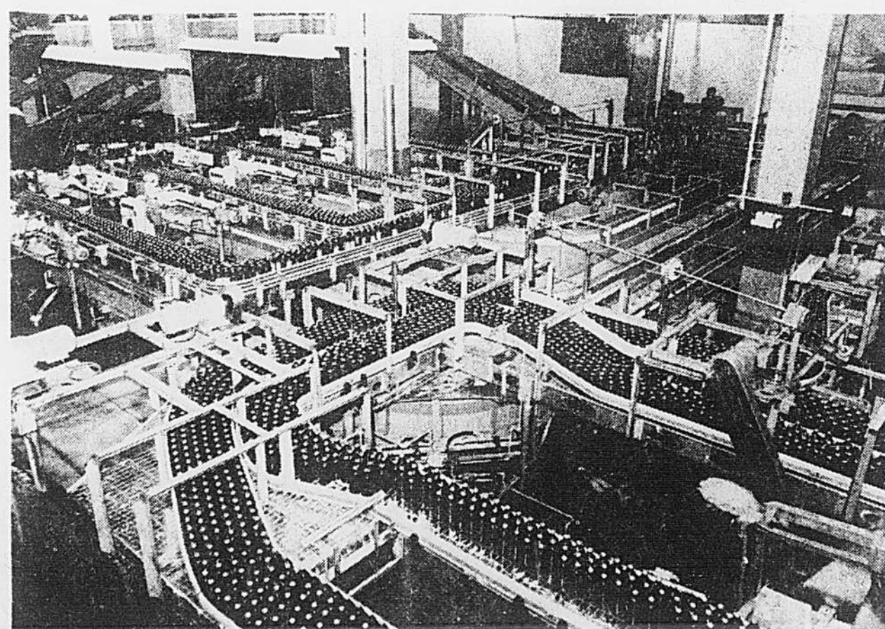
Vue partielle de la nouvelle chaîne d'embouteillage de l'usine montréalaise de la Brasserie Molson du Québec Limitée, inaugurée hier.
