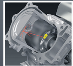
TRANSMISSION CVT RAFFINÉE LE CVT PERFECTIONNÉ LIVRE UNE MEILLEURE ACCÉLÉRATION À PARTIR DE L'ARRÊT ET UN FREIN MOTEUR PLUS EFFICACE.*
