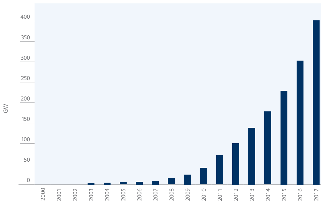
FIGURE 2 – ÉVOLUTION DE LA PUISSANCE SOLAIRE INSTALLÉE DANS LE MONDE (GW)
