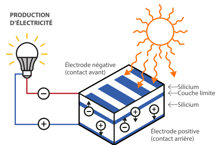
FIGURE 6 – L'EFFET PHOTOVOLTAÏQUE
