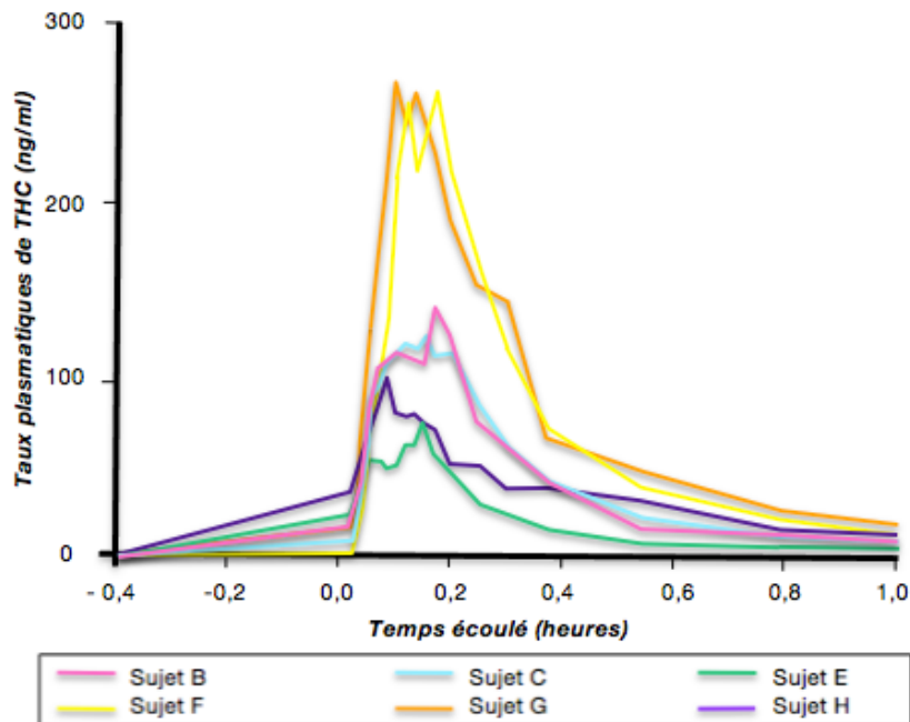
Figure 3 Concentrations plasmatiques de THC suivant la consommation contrôlée d'une cigarette contenant de 3,55 % de THC chez 6 sujets
