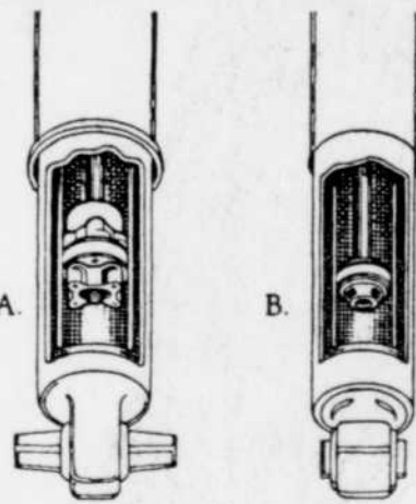
A. Amortisseur arrière de la 505 SR Peugeot et son imposant système de soupapes, qui lui permet de jouer un double rôle — pour le confort, et pour la tenue de route. B. En comparaison, amortisseur arrière de la Cadillac Seville.
