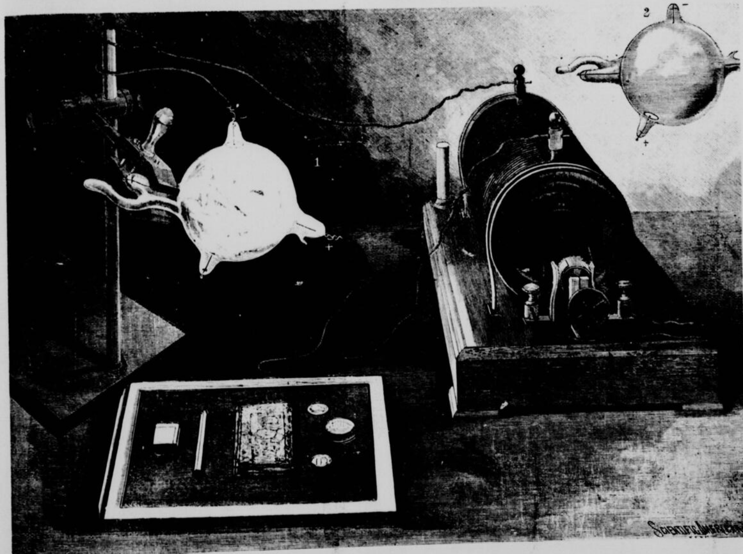
NOUVELLE DÉCOUVERTE PHOTOGRAPHIQUE. — APPAREIL DE WRIGHT POUR LA PHOTOGRAPHIE, SYSTÈME RENTGEN
