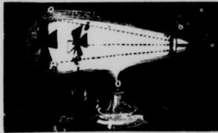
Fig. 1.—Tube de Crooke faisant voir l'ombre.
