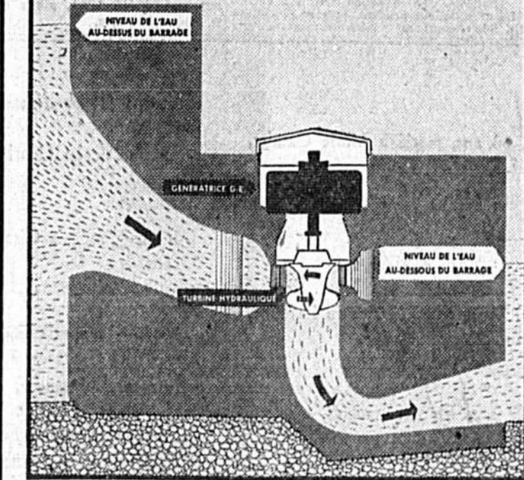
Croquis simplifié démontrant de quelle façon la force hydraulique sera transformée en électricité. Chaque génératrice sera actionnée par une turbine placée sur le trajet de l'eau traversant le barrage, du niveau supérieur au niveau inférieur du fleuve.
