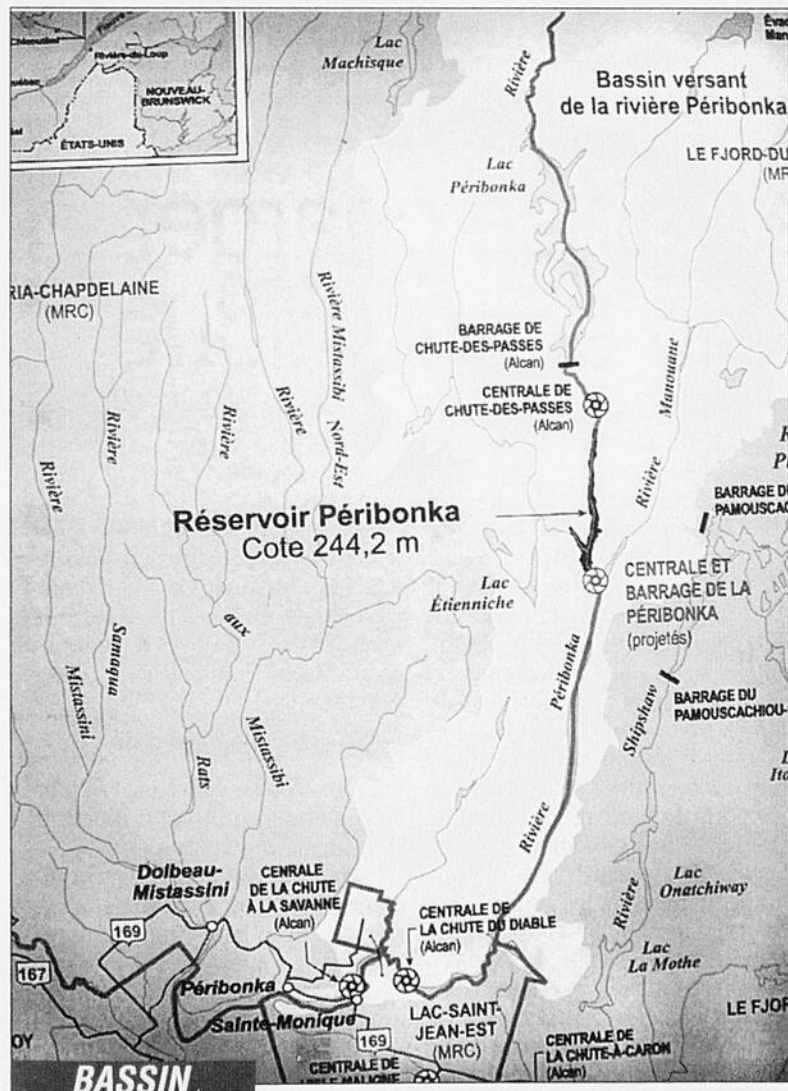
Cette carte montre l'aménagement du bassin de la rivière Péribonka où trois installations hydroélectriques sont en opération.
