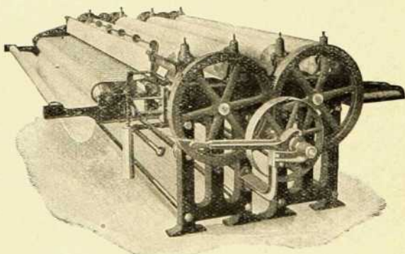
Calandre "Beaver" à 4 rouleaux.
