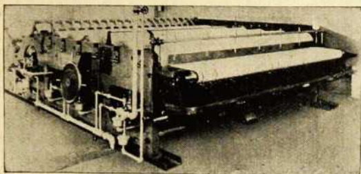
Représentant notre calendre "LONDON IMPERIAL" repassant et séchant des deux côtés d'une seule opération.
