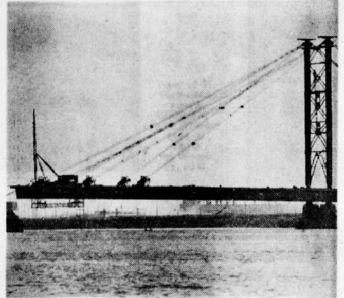
Suspendues par câbles à des pylônes temporaires, les sections du tablier s'aboutent...
