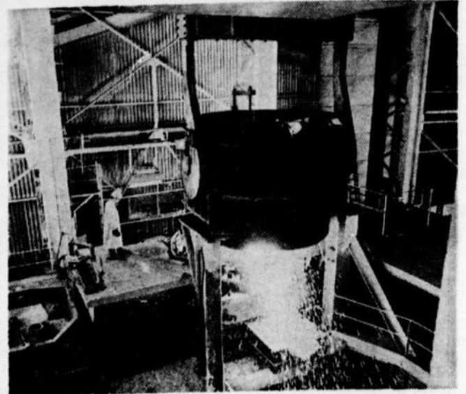
Amené de la fournaise dans un immense "pot" qui peut contenir 60 tonnes d'acier, le liquide en fusion en sort pour tomber dans le "bassin de coulée". De là, il se dirige sur une sorte de tremplin où il sera refroidi pour devenir une brame d'acier de longueurs variables.
