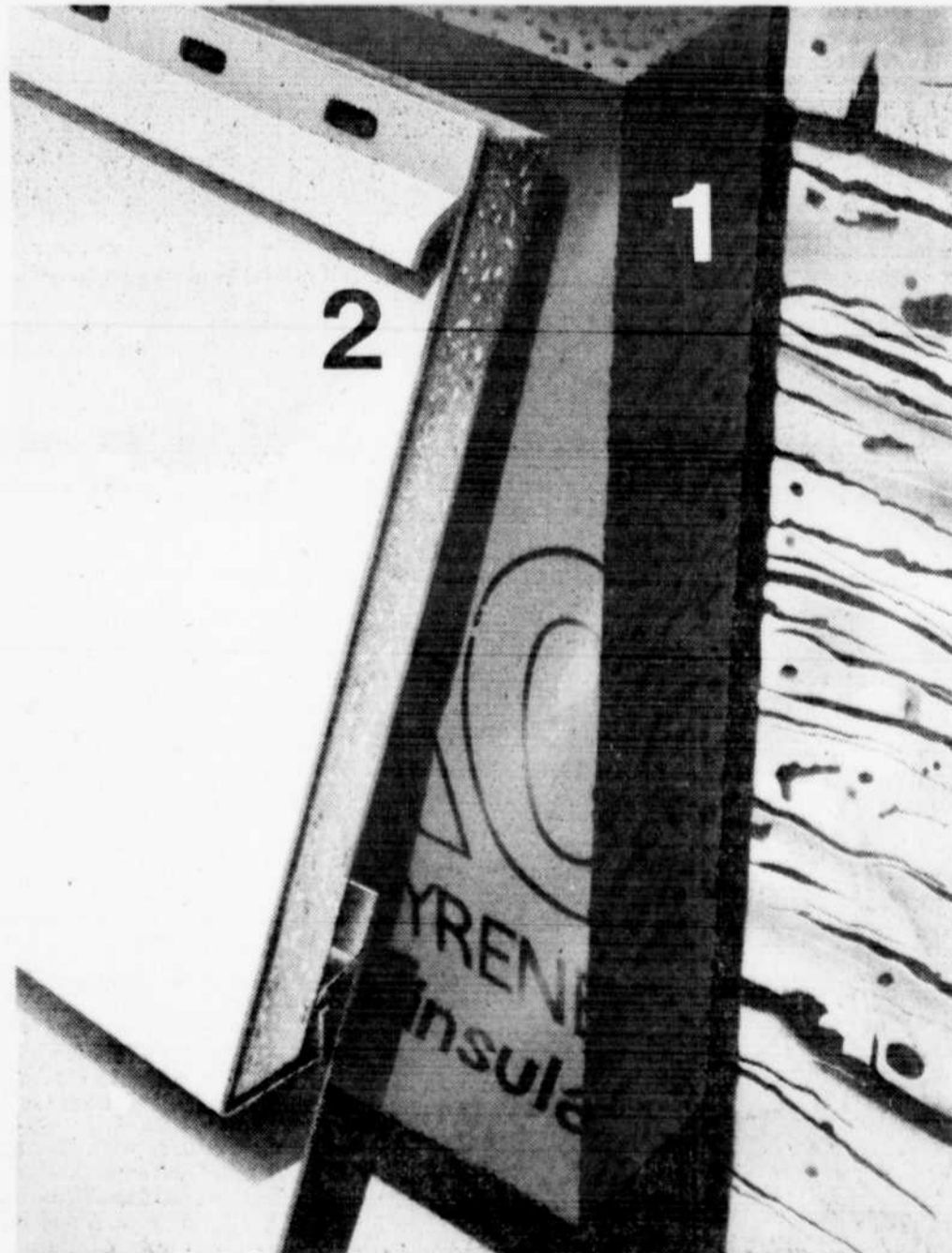
Les deux éléments constitutifs duo Alcan: revêtement-super isolant, la feuille isolante de Styrofoam SM en bleu (1), puis, à l'extérieur, le revêtement d'aluminium renforcé Alcan (2).
