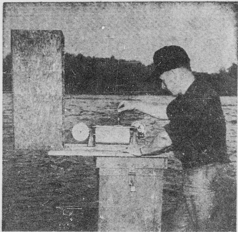
CINQUANTE MESUREURS, dont plusieurs sont automatiques, sont placés par les arpenteurs hydrographiques aux endroits stratégiques dans le secteur international du Saint-Laurent et sont vérifiés une fois par semaine afin de révéler le flot du fleuve et ses variations.
