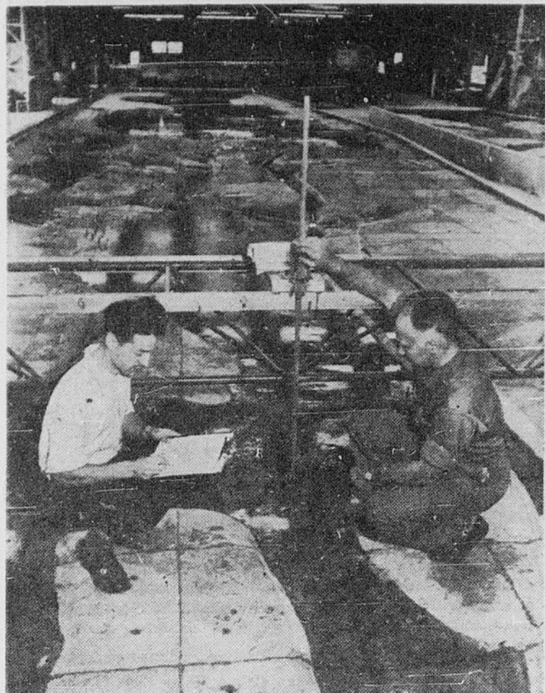
LES SPECIALISTES WOLF JENKNER (à gauche) et CLIFF DAVIDGE de l'Hydro d'Ontario mesurent les niveaux de l'eau sur le modèle numéro un de l'aménagement du Saint-Laurent à Islington. A l'aide d'un instrument de précision, soutenu par un "dolly", le mesurage se fait avec un jaugeage à point.
