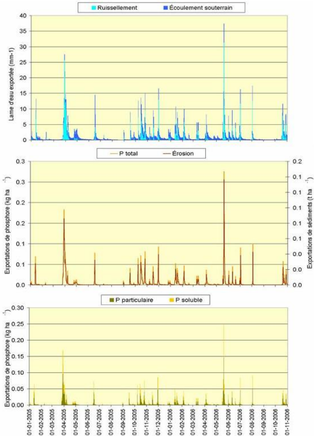
Figure 2. Séries chronologiques du ruissellement, de l'écoulement souterrain, des exportations de sédiments et des exportations du phosphore total, soluble et particulaire de janvier 2005 à novembre 2006 à l'exutoire du ruisseau au Castor
