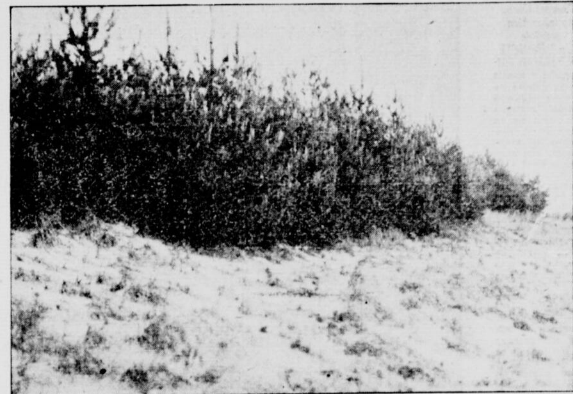
Ici, c'était déjà le désert. Pour sauver le sol envahi par les sables, on a planté des pins sur les dunes mouvantes. Et maintenant, une riche forêt en formation accomplit son magnifique travail de fécondité.
