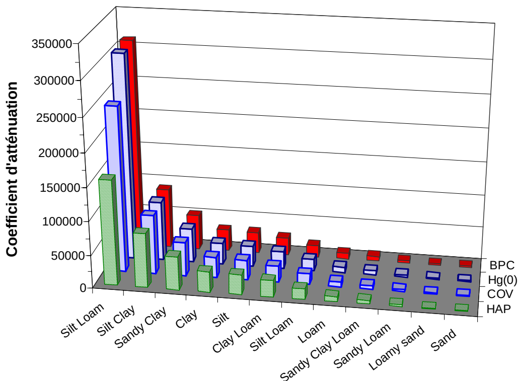
Figure 2. Coefficients d'atténuation pour l'intrusion de vapeurs estimés pour 12 types de sol et 4 substances selon le modèle JEM
