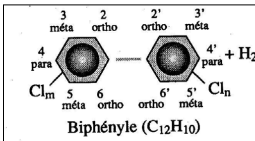
Figure 1. Structure du noyau de base des BPC
