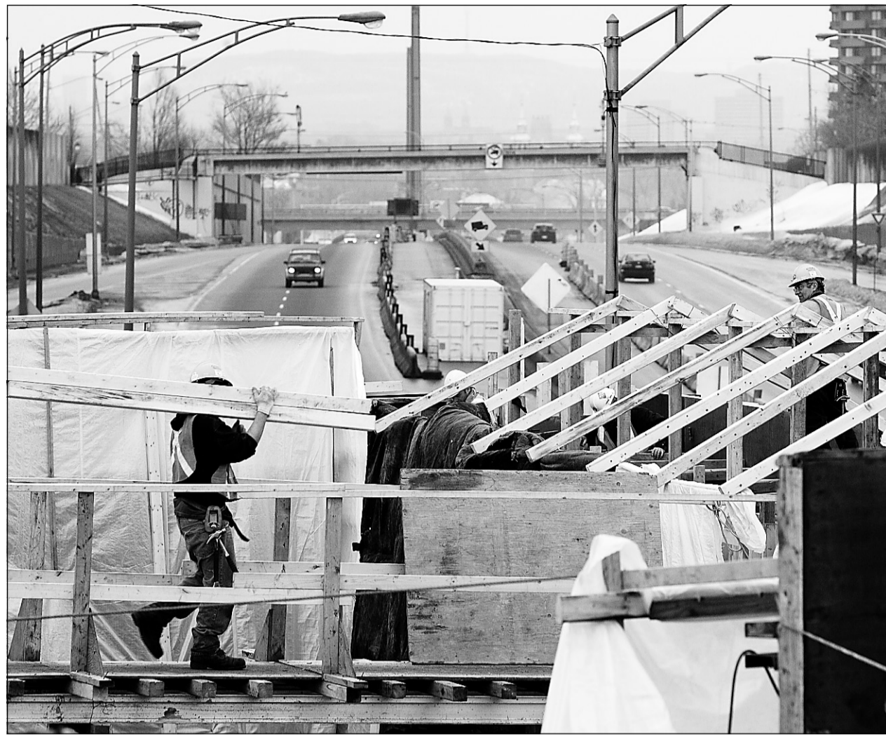
Des travailleurs s'affairent depuis le début du mois de mars à rebâtir la structure du viaduc du boulevard de la Concorde, qui s'est effondré l'automne dernier. Quinze structures possédant des caractéristiques similaires devraient faire l'objet de travaux de consolidation au cours des cinq prochaines années.
