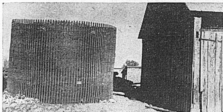
Voici le silo portatif Rosco à 3-sections dans lequel Johnnie-Boucher emmagasine de 32 à 35 tonnes d'ensilage de blé d'inde pour son bétail à tous les automnes.
