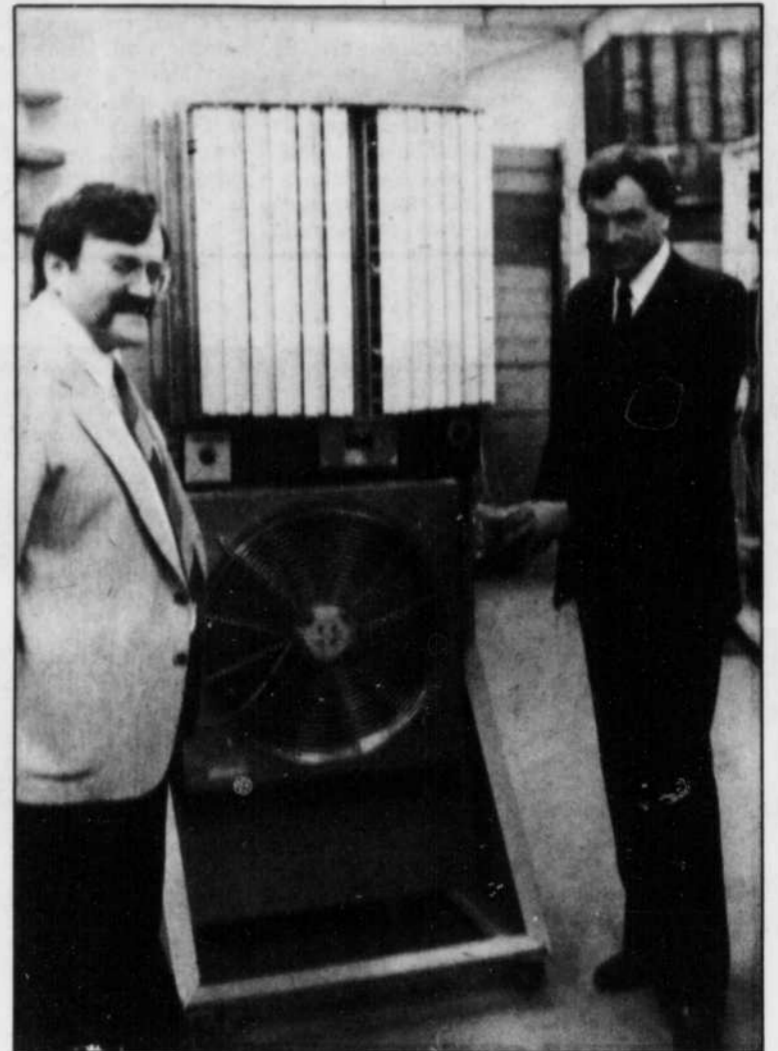
M. Claude Caron, vice-président d'Aston Industries, est heureux de montrer au commissaire industriel du COPERS, M. René Bérubé, le tout nouvel appareil fabriqué par sa compagnie, soit un échangeur d'air à vitesse variable.
