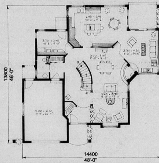
Rez-de-chaussée: 113,13 m 2 (1257 pi 2 )
