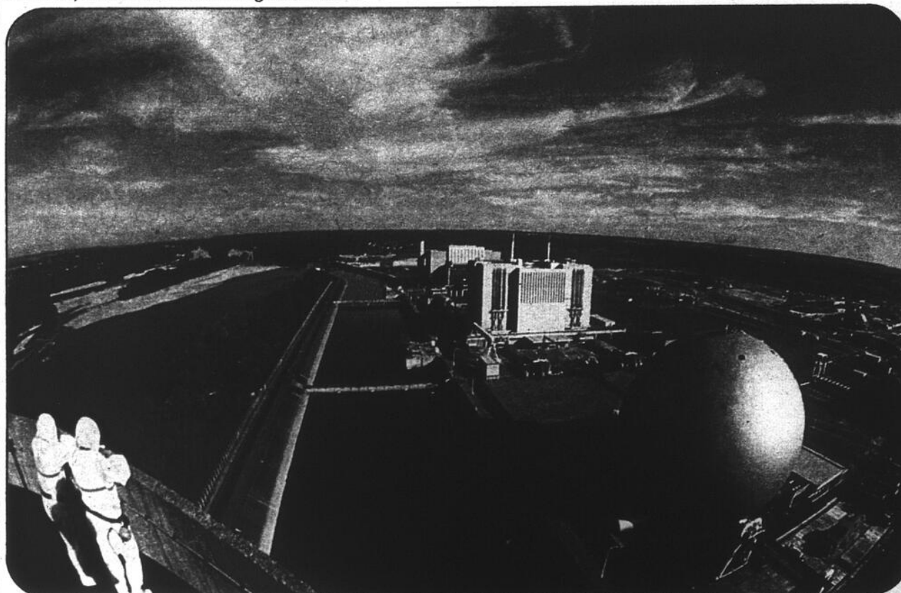
Vue extérieure de la centrale nucléaire de Chinon, en France, montrant l'édifice du réacteur, au centre, au bord d'un canal longeant la Loire.
