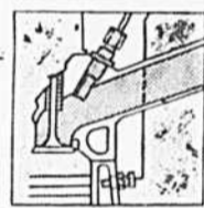
Injection d'essence au lieu d'un carburateur.
