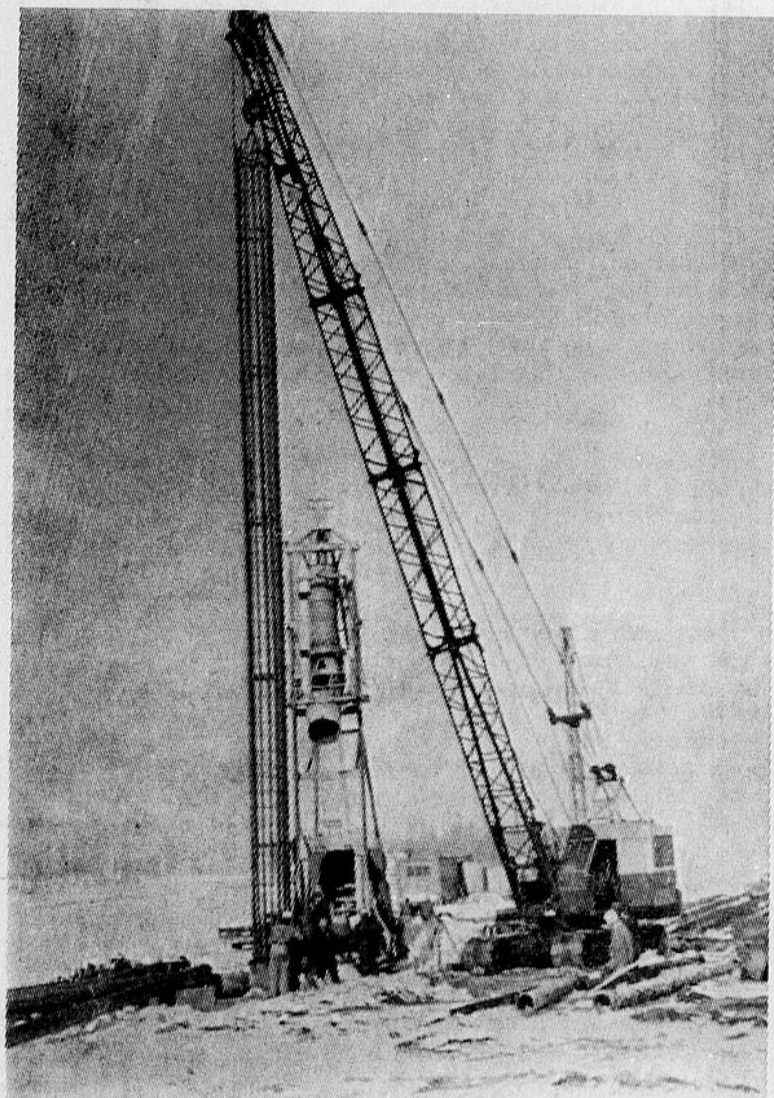
AU VIADUC DE LA ROUTE 41. — Un nouveau genre de fondation est effectué par les Entreprises Petrifond en regard de la construction du viaduc de la route 41. Ce nouveau mode d'opération consiste à introduire dans le sol des tuyaux d'acier jusqu'à ce qu'ils touchent le roc c'est-à-dire jusqu'à plus de 300 pieds parfois de profondeur. Dans ces tuyaux sont introduits des colonnes d'acier d'une longueur de 60 pieds et dont nous voyons la reproduction sur la photo ci-dessus.
