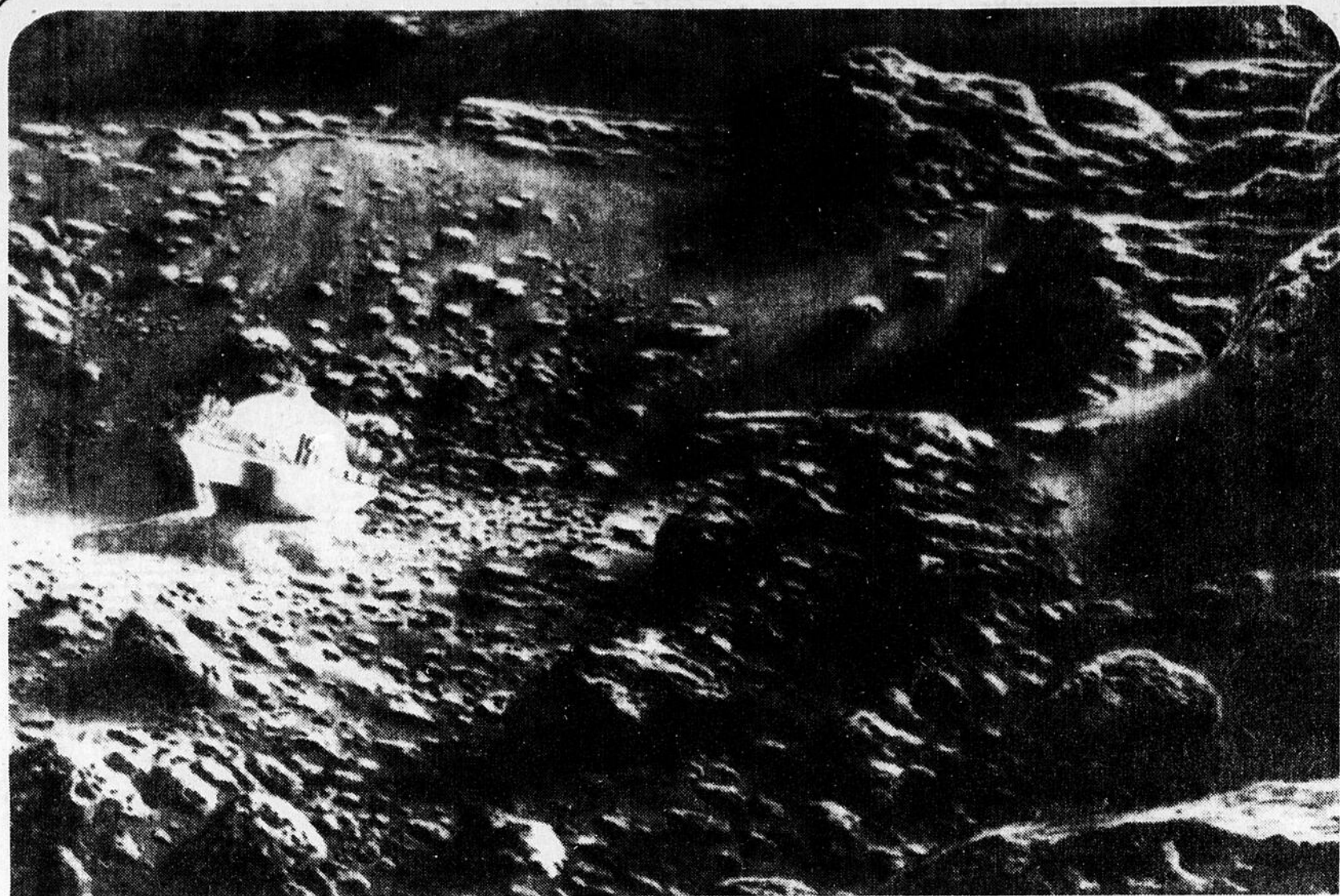
SONDE SUR LA SURFACE DE VENUS — Une sonde minuscule repose sur la surface de Venus, telle que vue par un artiste de la NASA. Ce n'est là qu'une des trois sondes identiques qui se sont posées sur Venus après avoir traversé son atmosphère hostile, sur la face de la planète s'opposant à la terre. Chacune des sondes transportait trois instruments spécialement conçus pour mesurer les conditions de l'atmosphère entourant Venus.
