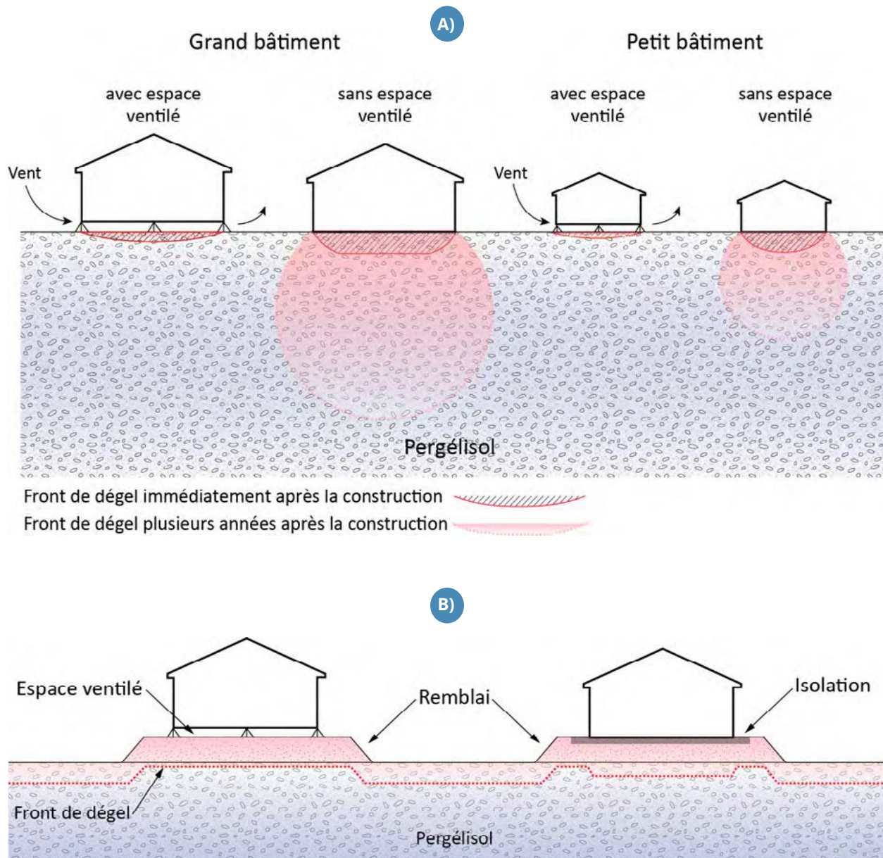
FIGURE 5.55 : A) POSITIONS DU FRONT DE DÉGEL SOUS DES BÂTIMENTS CHAUFFÉS EN FONCTION DE LEUR DIMENSION, DU TYPE DE FONDATION ET DU TEMPS. B) DEUX TYPES DE SYSTÈMES DE FONDATION QUI REPOSENT SUR UN REMBLAI GRANULAIRE.
