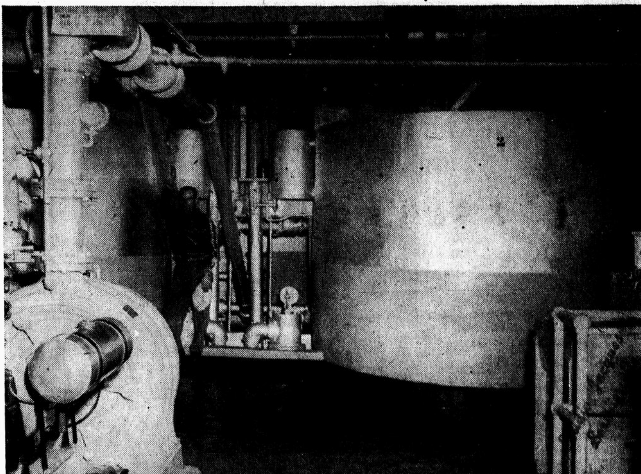
Cette photo nous montre les deux réservoirs-filtres et au centre les contrôles.
