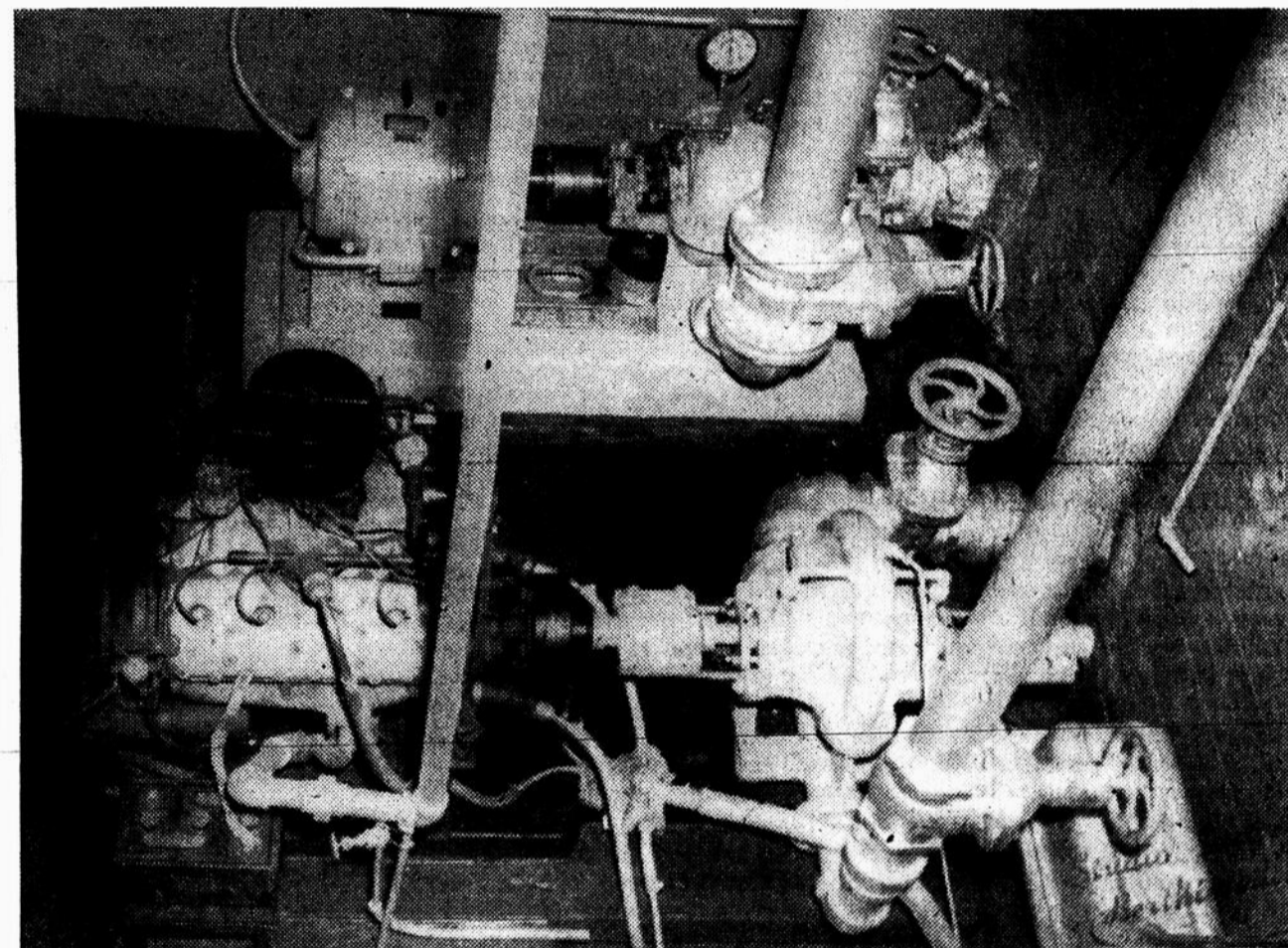
Au fond, la pompe électrique qui tire l'eau du fleuve. En avant, la pompe d'urgence, mue par un moteur à gasoline, qui peut remplacer l'autre quand l'électricité manque.
