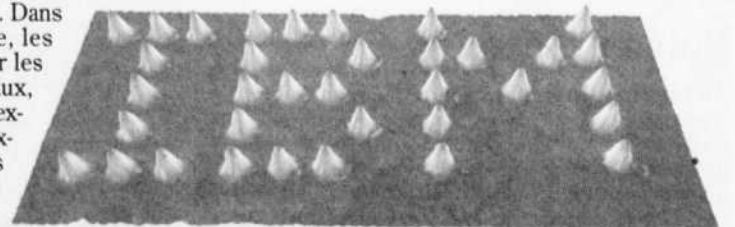
Le commencement, une œuvre des chercheurs Eighler et Schweitzer en 1990: 35 atomes de xénon sur une plaque de nickel à -270 degrés Celsius.
