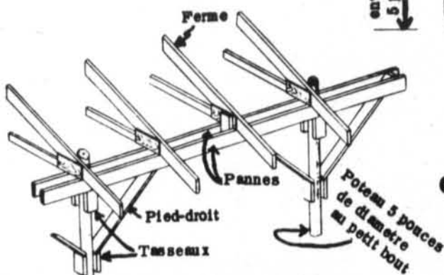
Figure 111 Charpente typique Haut de mur et toit
