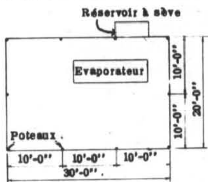
Figure 1 Sucrierie sur poteaux (Vue en plan)
