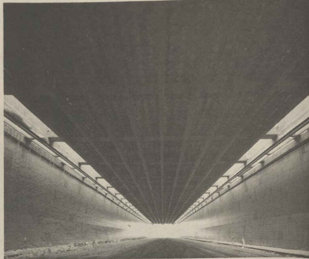
A chacun des portails, un brise-soleil formé d'avéoles d'une profondeur de 24 pouces atténué progressivement la lumière du jour pour passer à une intensité de douze pieds-bougies, 1,000 pieds à l'intérieur du tunnel.
