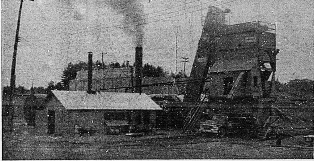
Photo du nouveau plan d'asphalte de la Compagnie d'Asphalte et de Pavage Laurentienne Ltée, dont M. Anatole Desjardins de Ste-Thérèse est le président et M. Simon Latour de St-Jérôme est vice-président et gérant général. Ce plan est situé à l'ouest de l'autoroute de St-Jérôme. Ce plan a coûté environ $250,000.00 et peut fournir 200 tonnes d'asphalte à l'heure. Une vingtaine d'hommes travaillent à ce plan. C'est encore une nouvelle industrie pour St-Jérôme.
