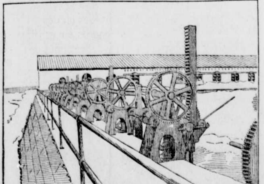
Vue de l'emboclement servant à régler le niveau de l'eau.
