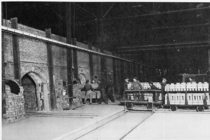
Afin de répondre à la demande croissante, des entreprises anciennes se modernisent : chargement des fours de la briqueterie de La Prairie. Deux ensembles de fours sont chauffés au charbon et troisième l'est au gaz. (Société historique de Laprairie de la Magdeleine)
