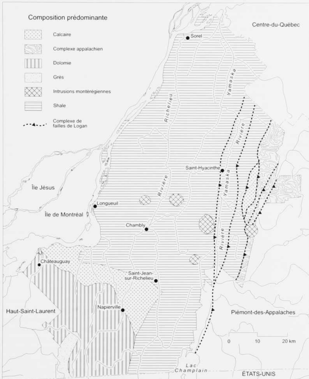
Carte 2 La géologie
