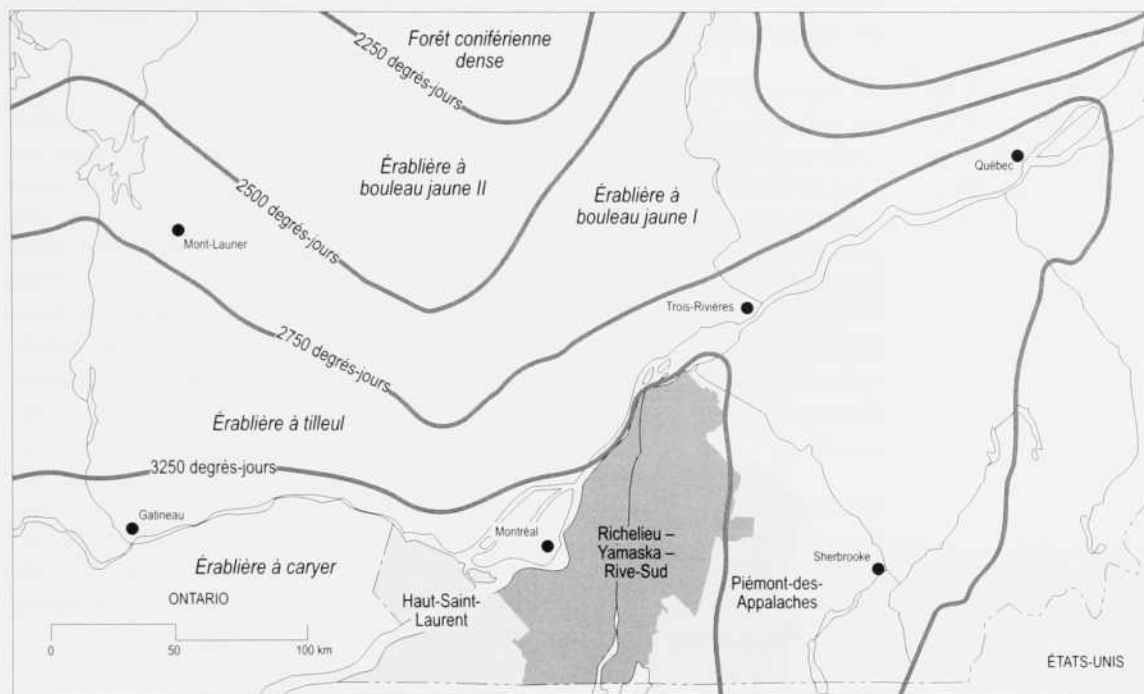
Carte 6 Le bilan radiatif et les végétations dominantes
