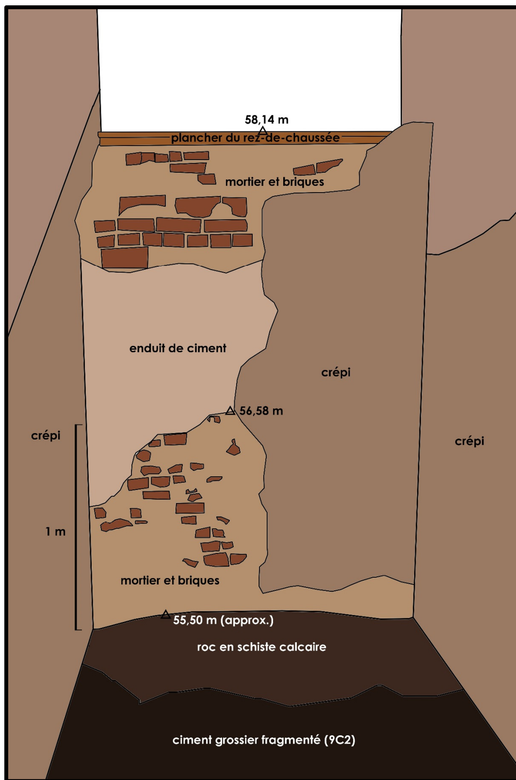
Figure 65. Croquis du parement sud du mur 9C100 (Dessin : S. Noël).
