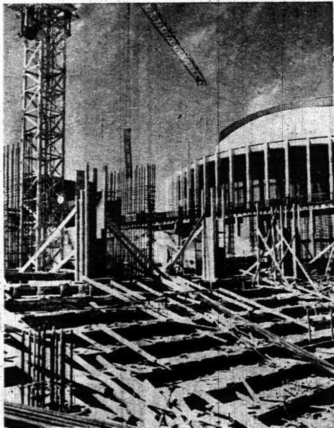
UN THEATRE S'ELEVE — Deux mois à peine après le début des travaux de construction de l'édifice des théâtres, à la Place des Arts, la structure dépasse déjà le niveau de la rue, soit une hauteur d'une cinquantaine de pieds du sol. Outre les fondations, les deux-tiers de la charpente de béton armé du Théâtre Port-Royal (800 places) ainsi que le tunnel des services mécaniques sont déjà terminés. Des équipes d'ouvriers travaillent six jours par semaine sur le chantier de façon à parachever les travaux pour le 1er avril 1967.
