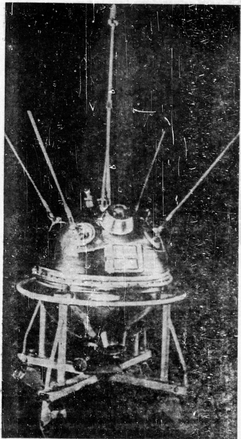
VOICI LA PHOTO OFFICIELLE DE "LUNIK" — La Pravda a publié récemment la première photo officielle du principal élément de la "planète artificielle soviétique" lancée le 2 janvier. Il s'agit d'une sphère pesant 361 kilos équipée de 4 antennes au milieu desquelles est placé un long tube dont l'extrémité est constituée par un instrument pour détecter le champ magnétique lunaire.
