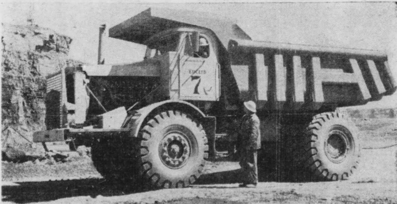
CAPACITE AUGMENTEE — La caisse d'aluminium de ce gros camion employé dans les carrières permet d'augmenter de QUATRE TONNES la capacité de transport du véhicule. Cette caisse du
