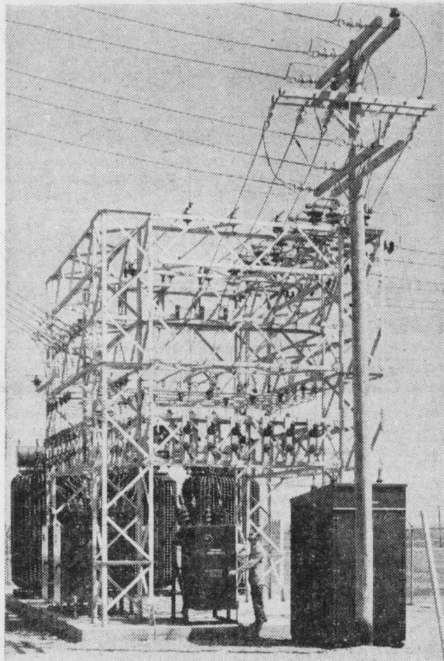
CETTE SOUS-STATION, érigée sur la rue Volta à Arvida, est l'une des plus modernes que possède actuellement la Compagnie Electricque du Saguenay. Elle constitue, comme tant d'autres, le centre nerveux du système de distribution d'un quartier, d'une ville, d'un village de notre région.
